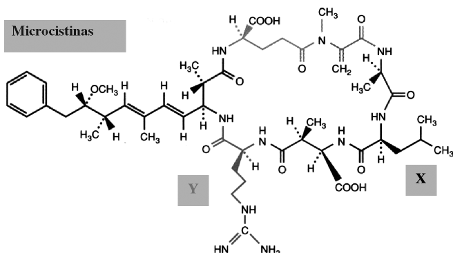
Fig. 1. Estructura química de las microcistinas (Mcs).
